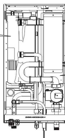
Papildomas el.šildytuvas
