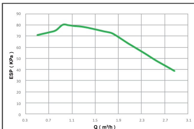
Vidaus blokas 160
